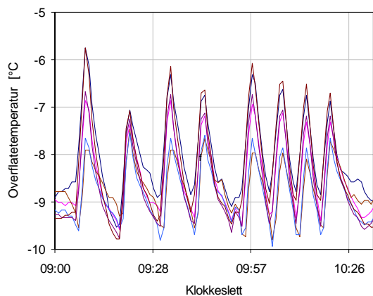
Figur 16. Registrerte overflate-temperaturer på skinnkjølerens teflonbånd gjennom en tre timers periode. Gjentatte gjennomløp av målesonder fordelt over båndets bredde. Målinger gjengitt med tillatelse fra Fiskeindustriens forskningsinstitutt, Island (RF).
