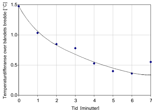
Figur 17. Beregnet stigning i båndtemperatur over båndets bredde. Tidspunkt '0' refererer til kjølerens innmatingsende. Grafen bygger på samme temperaturdata som ligger til grunn for figuren her til venstre.
