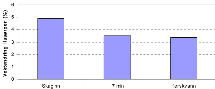
Figur 38. Det totale utbytte fra trimmet filet til skinet filet.
