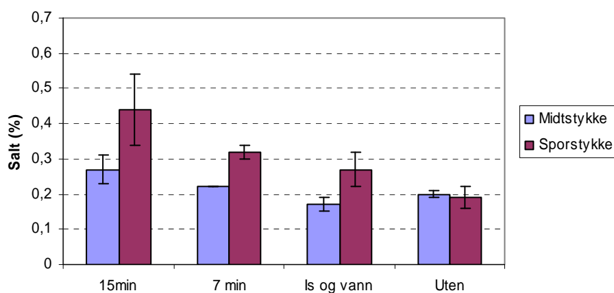
Figur 42. Målt saltinnhold i muskelen ut fra Skaginn-linjen etter lakeopphold i 15 min, 7 min og 15 min med kun is og vann, samt prøve uten lakedypp. Målinger er gjort både i midtstykket og i sporden. Saltinnholdet i laken ble målt til 2,3 % salt.
