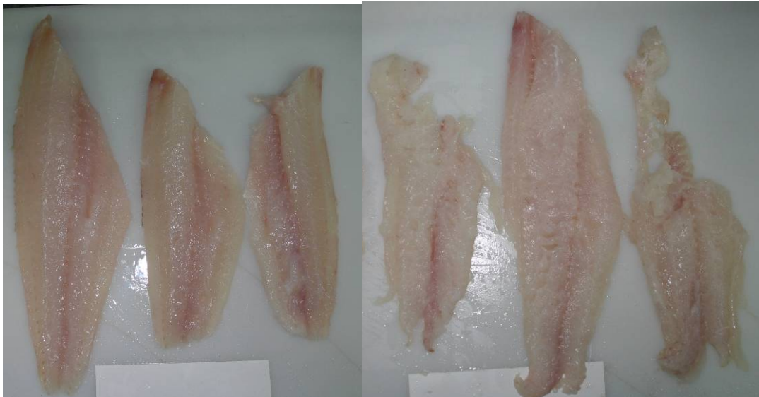
Figur 23. Filet etter skinning av ca. 180 g hysefileter. Skaginn til venstre og Baader 51 til høyre.
