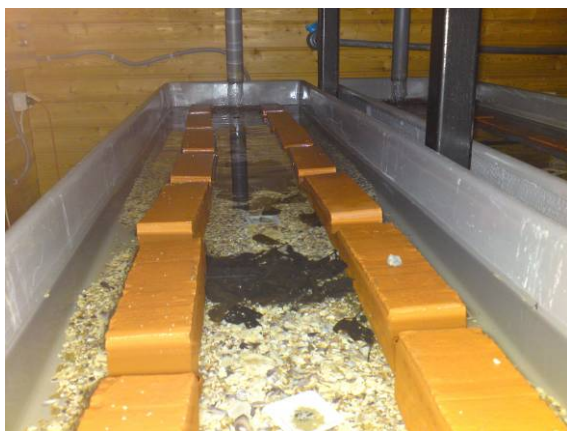
Bilde 4a og b Viser forsøksoppsettet i lengdestrømsrenner og utføringskammer
