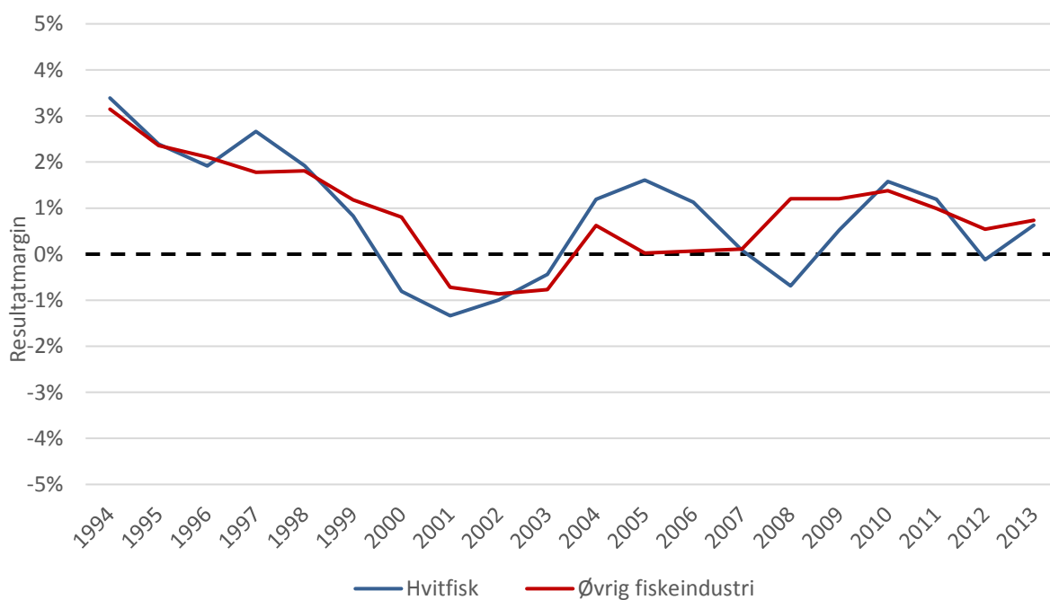
Figur 7 Resultatmargin i hvitfiskindustrien og i øvrig fiskeindustri. Ordinært resultat før skatt og tap/gevinst på valutasingring/valutahandel i prosent av omsetning. Tre-års sentrert veid gjennomsnitt.
