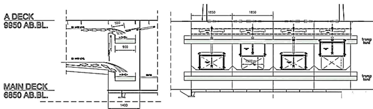
Figur 1 Skisse av mottaksbinge
