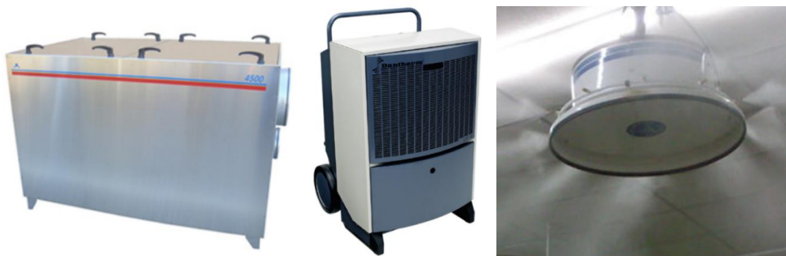
Figur 10 Industriell avfukter (t.v.), mobil avfukter (midten) og tåkesystem (t.h.) for henholdsvis reduksjon og økning av relativ fuktighet i lager.
